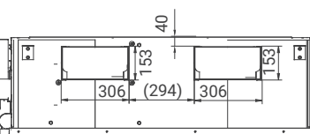
Схема отверстий для выхода воздуха
